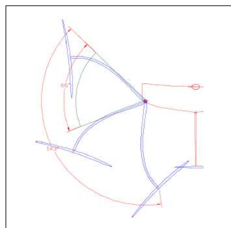
La cinématique des Foils
